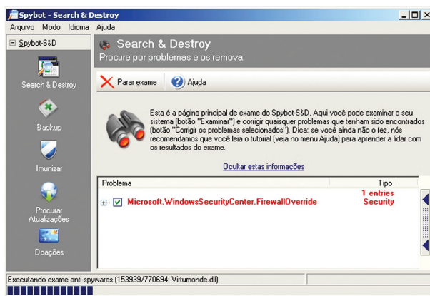
Figura 7.3: Varredura
