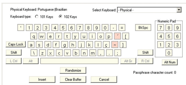
Figura 5.4: Teclado virtual
