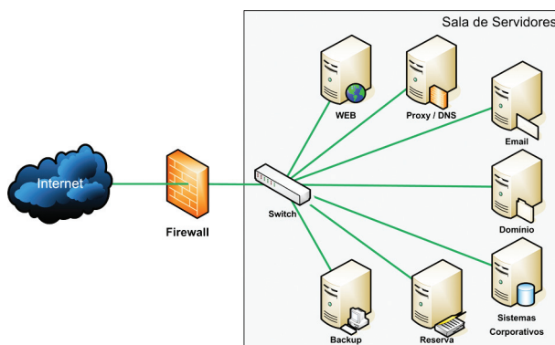
Figura 7.7: Firewall corporativo
