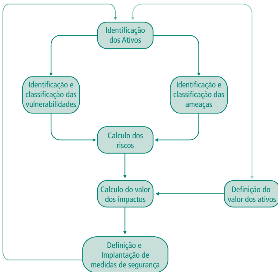
Figura 2.5: Ciclo da Segurança da Informação
