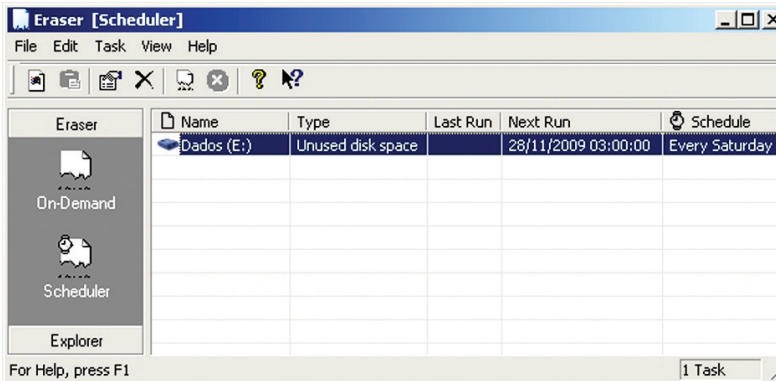
Figura 6.7: Agendamento completo
