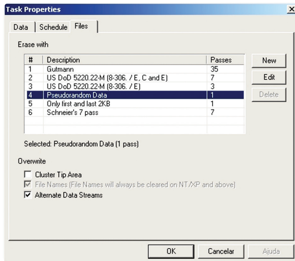
Figura 6.6: Guia Files
