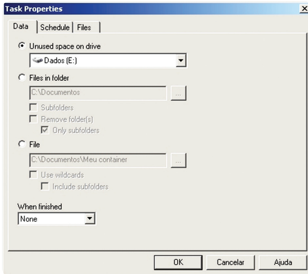
Figura 6.3: Guia Data
