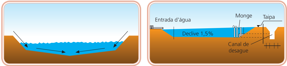
Figura 3.10: inclinação no centro (esquerda) e declividade no tanque (direita)
