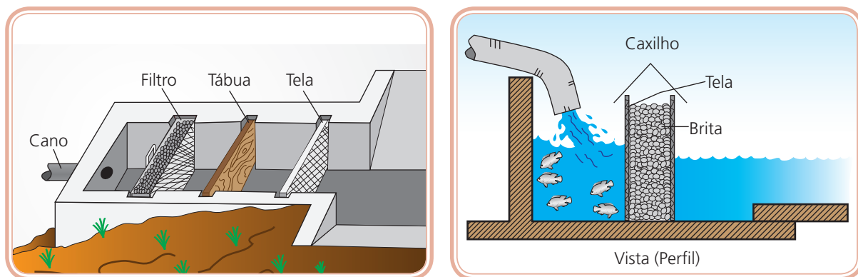
Figura 3.8: filtro em tanques de alvenaria (esquerda) e filtros em canais de abastecimento (direita)
