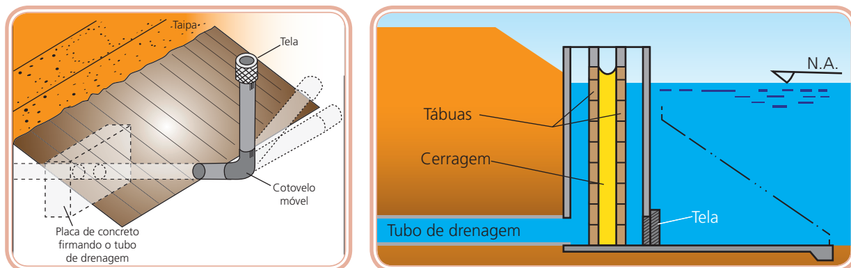
Figura 3.9: Tipo cotovelo (esquerda) e tipo monge (direita)
